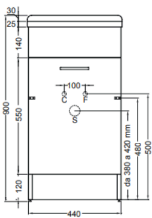
VISTA FRONTALE
