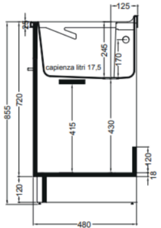
SEZIONE A-A'
