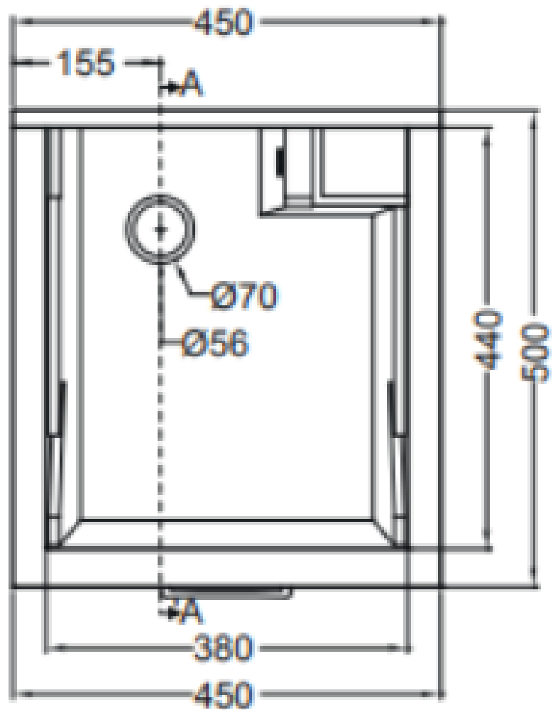
PIANTA
